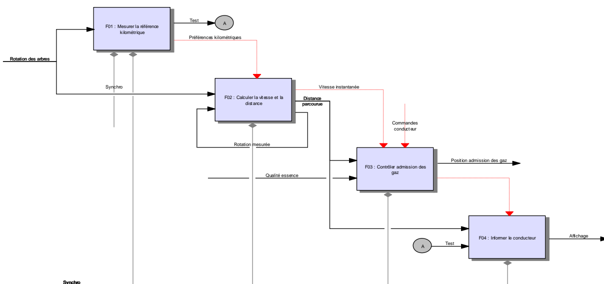
Diagramme SADT
